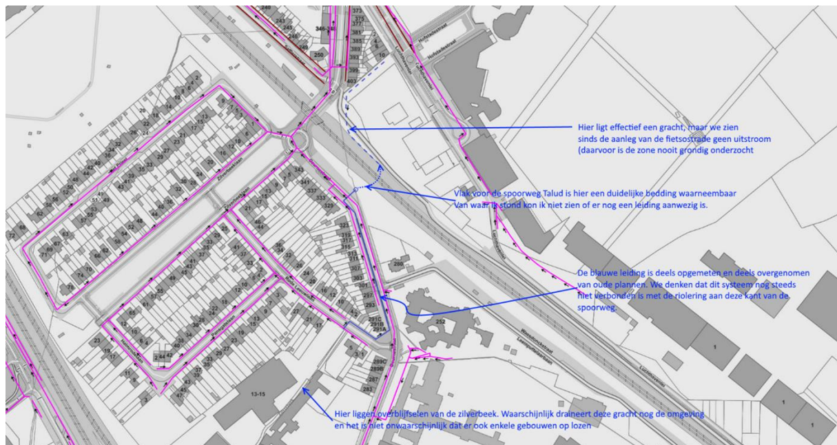
Figuur 5. Lijn 27: Het is mogelijk dat hier ook nog een duiker onder de spoorlijn zit. Onze gegevens zijn zeer onvolledig. In het hemelwater- en droogteplan van Mortsel is er niet voorzien dat deze kruising nog bruikbaar zou zijn. Qua reliëf is het ook moeilijk om vanaf deze locatie nog een waterloop te bereiken. Indien de kruising nog bestaat kunnen we wel bekijken of ze een rol kan spelen in het lokale watersysteem.
